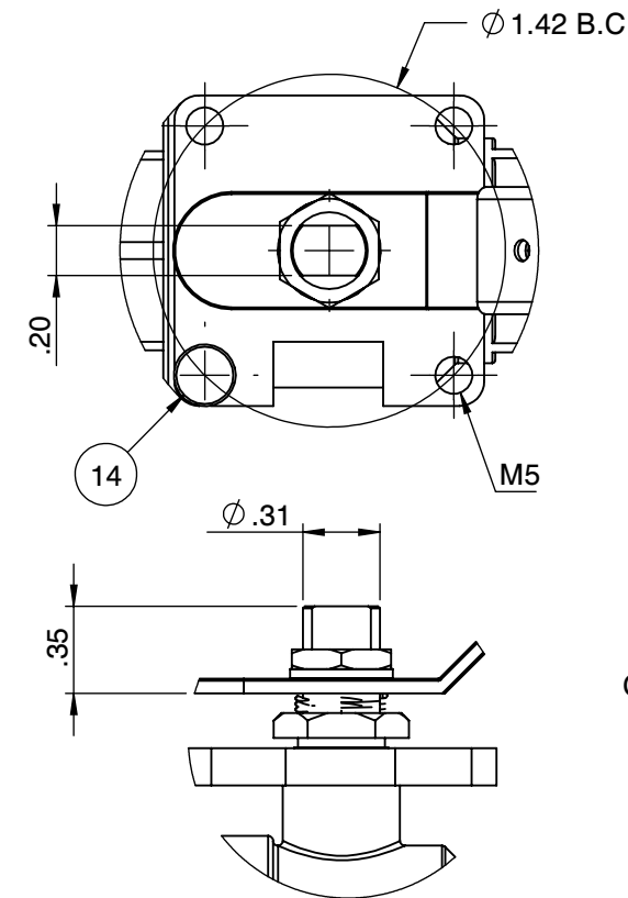
Actuator ISO Mounting Flange (F04)
