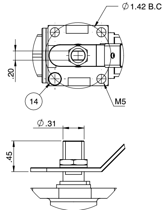
Actuator ISO Mounting Flange (F04)
