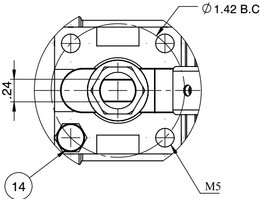
Actuator ISO Mounting Flange (F04)
