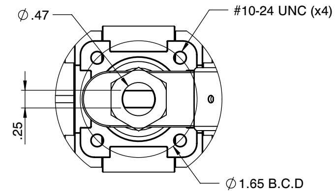
Actuator ISO Mounting Flange (F04)
