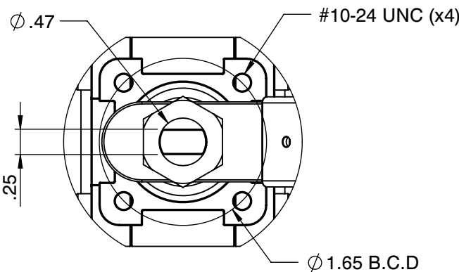
Actuator ISO Mounting Flange (F04)
