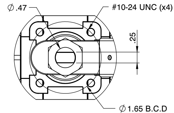
Actuator ISO Mounting Flange (F04)
