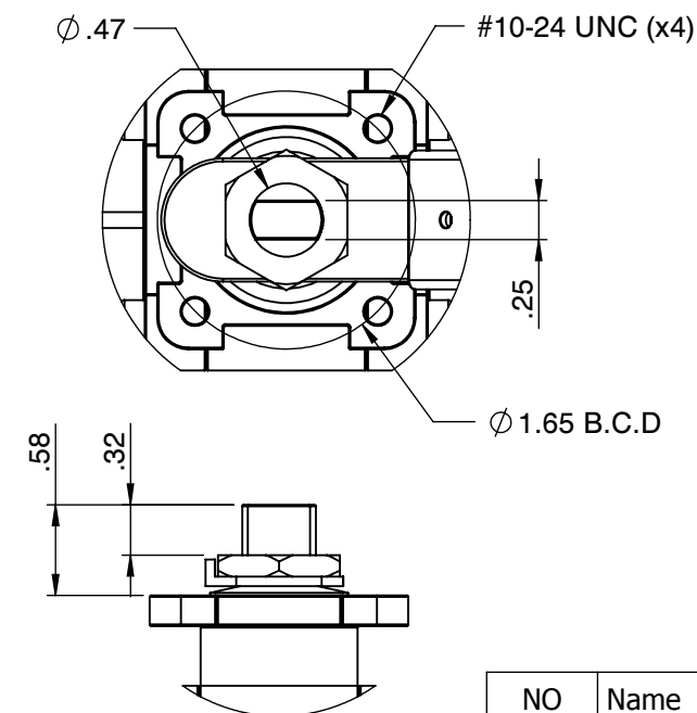
Actuator ISO Mounting Flange (F04)
