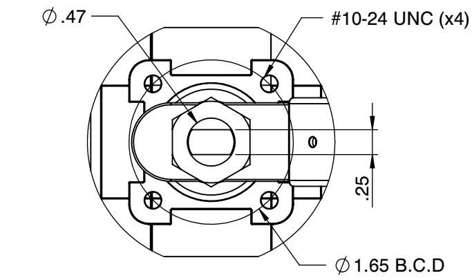
Actuator ISO Mounting Flange (F04)
