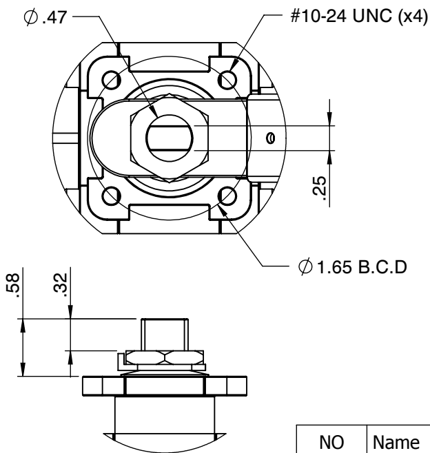
Actuator ISO Mounting Flange (F04)
