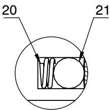
DETAIL : A DETAIL : B
