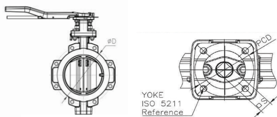
Lug Type BL631 BL731
